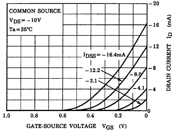
I_D - V_{GS}
